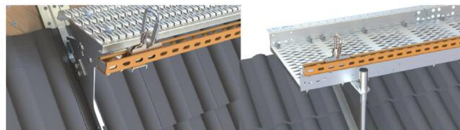
C-Schiene 250
